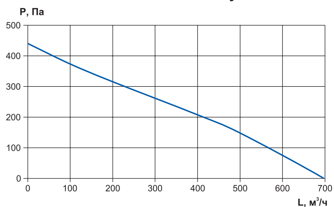
CV-SH-250-AC Grey
