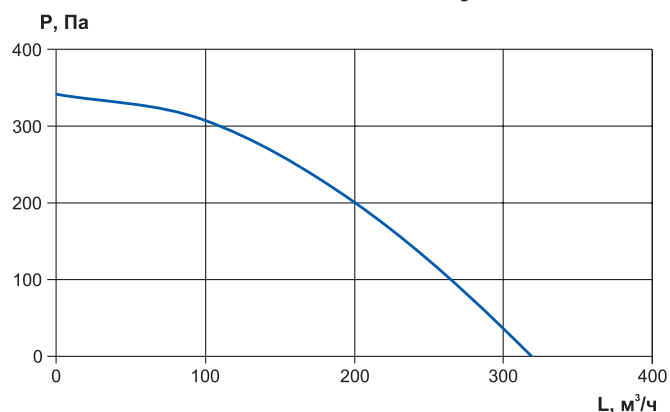
CV-SH-160-AC Grey
